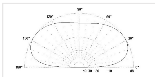
Vyzařovací diagram v rovině E
