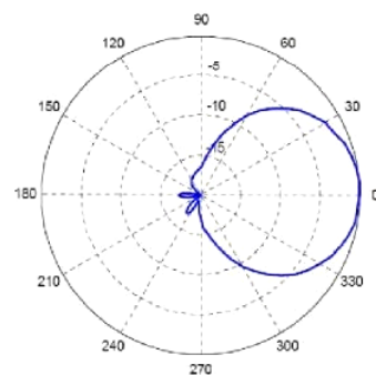
Vyzařovací diagram v rovině H (925 MHz)
